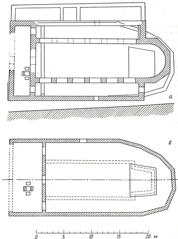
Рис. 1 — a — остатки двух базилик в Питунте (по И. Н. Цицишвили); б — реконструкция древнейшей базилики Питунта
