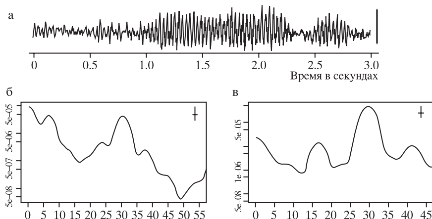
Рис. 4. Электрическая активность эмбриона рачка Artemia salina и периодограммы, характеризующие разные этапы его развития: а – электрическая осцилляторная активность эмбриона, калибровка – 20 мкВ; б, в – периодограммы, характеризующие электрическую активность эмбриона в разные периоды развития: на второй ( б ) и на шестой ( в ) день эмбриогенеза. Обозначения как на рис.1 б .
